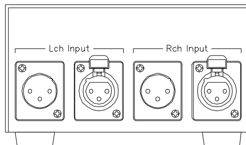
信号入出力部
